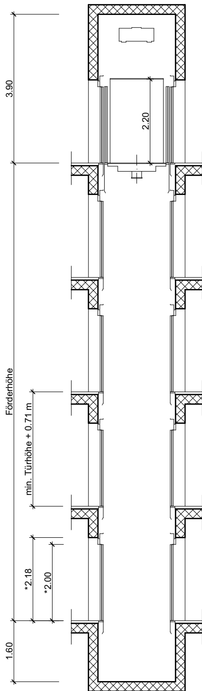
Türhöhe 2.00 *Option Türhöhe 2.10 = Türaussparung 2.28
